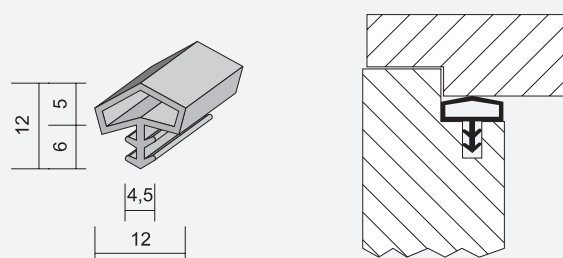
P110 | Dihtung za dovratnik
