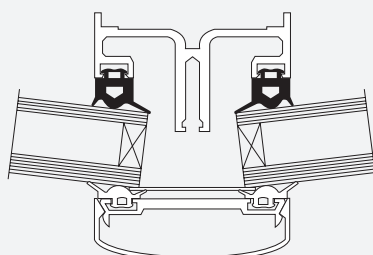
Tesnilo za fasadno notranje
