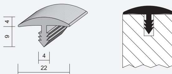
P114 | Odbojnik za stolove
