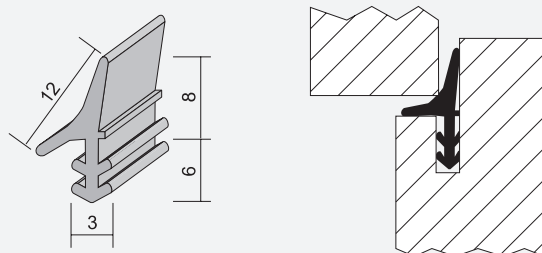
P115 | Dihtung za klizna vrata
