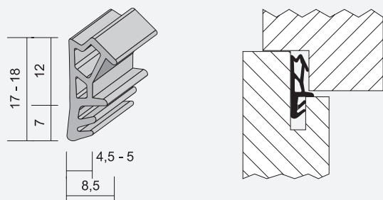
P113 | Dihtung za prozor
