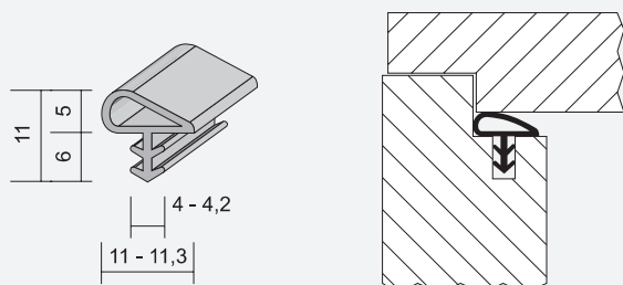
P109 | Dihtung za dovratnik
