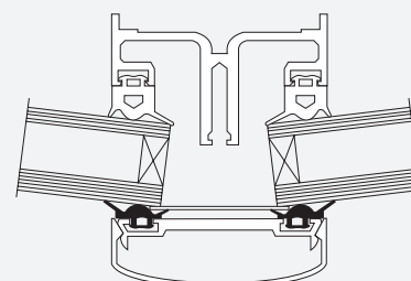
Zunanje tesnilo za zasteklitev
