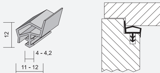
P112 | Dihtung za dovratnik
