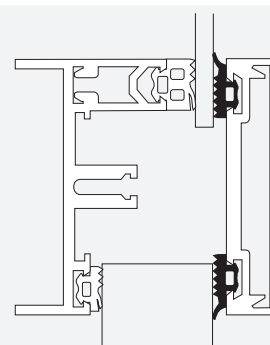
Zunanje tesnilo za zasteklitev
