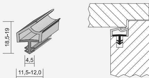
P116 | Dihtung za dovratnik
