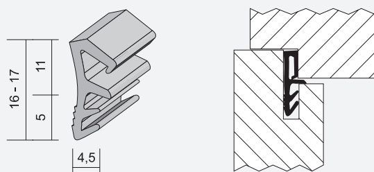
P111 | Dihtung za dovratnik prozora
