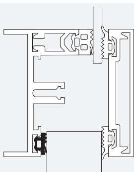
Notranje tesnilo za zasteklitev
